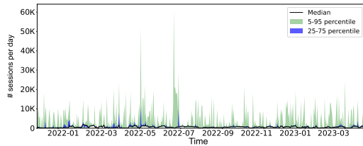
(d) CMD
